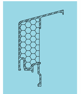
Aluminiumprofil mit Wärmedämmung
